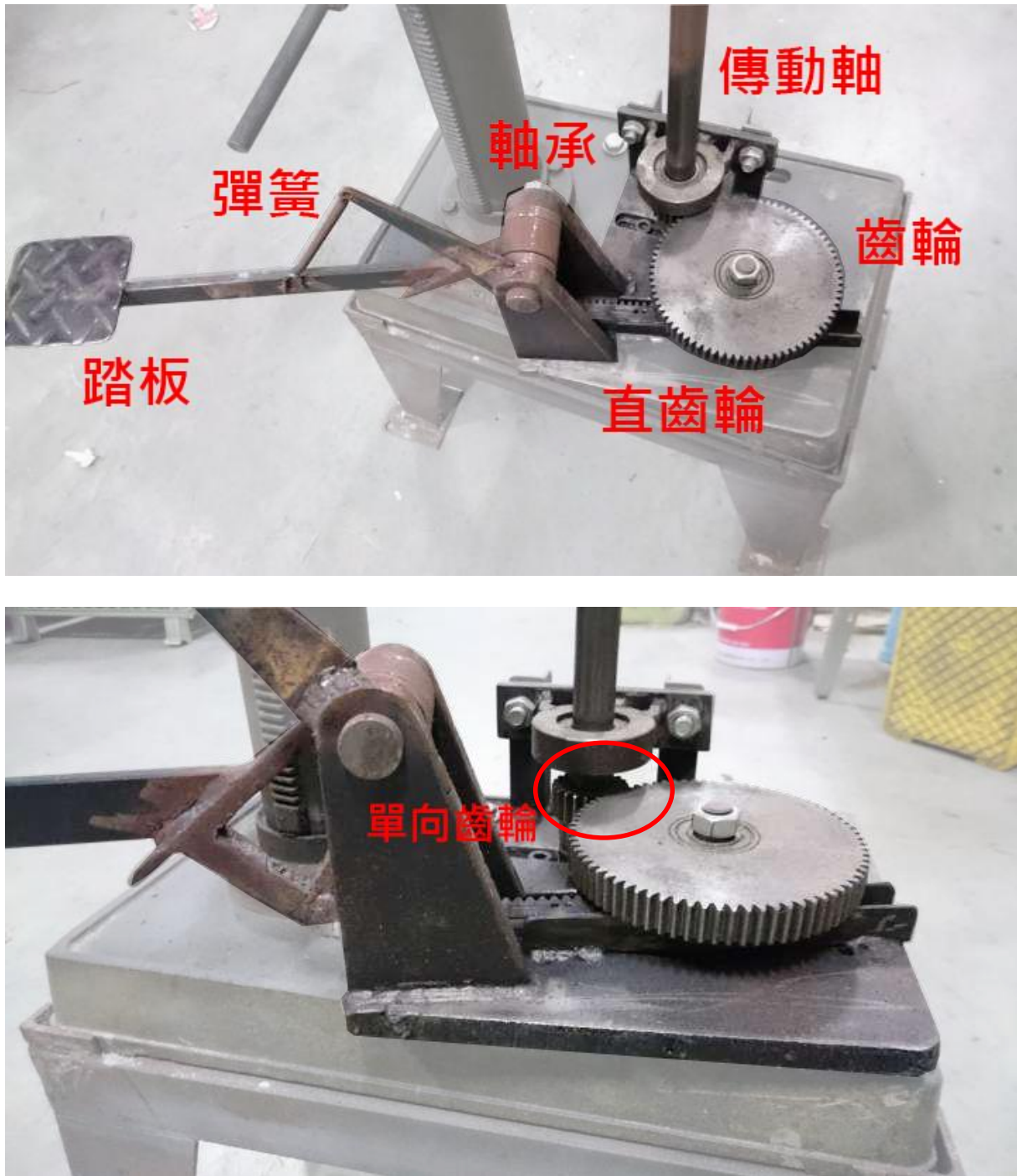
圖 11 腳踏動力鑽床傳動機構說明
